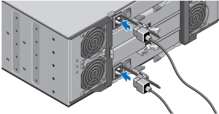
Αριθμός 4. Σύνδεση των καλωδίων τροφοδοσίας
